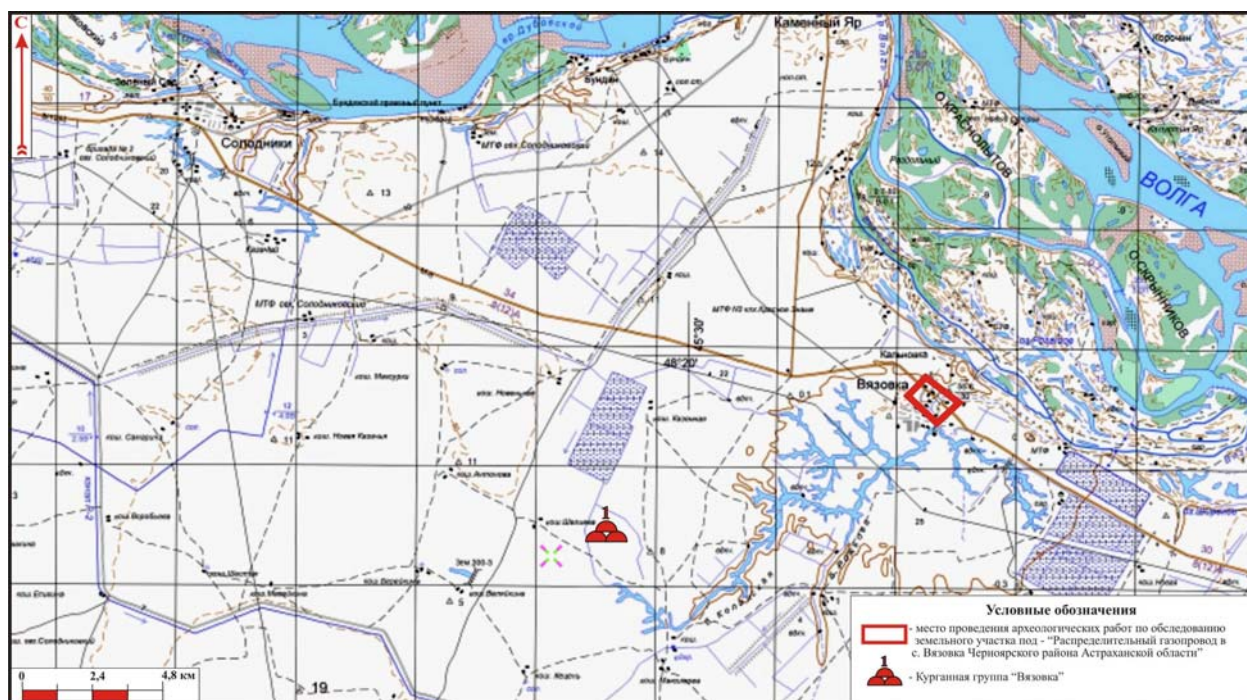
Илл. 3. Расположение земельного участка, отводимого под - «Распределительный газопровод в селе Вязовка Чернырского района Астраханской области», подлежащего археологическому обследованию, на местности, с указанием ОКН (памятников археологии), известных по архивным данным. Топографическая карта.
